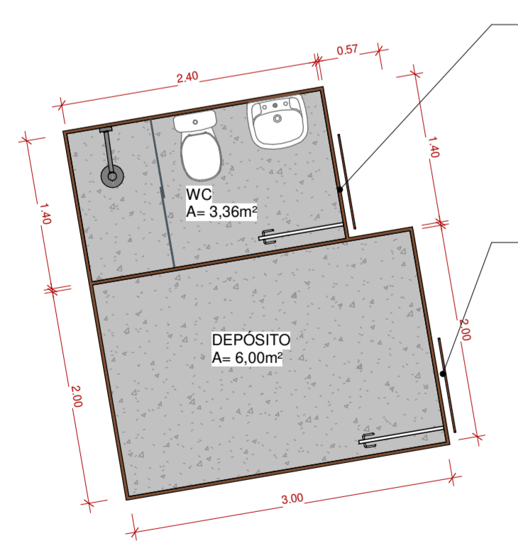
0.11 CANTEIRO DE OBRA - Chamada de detalhe 1 1 : 50
