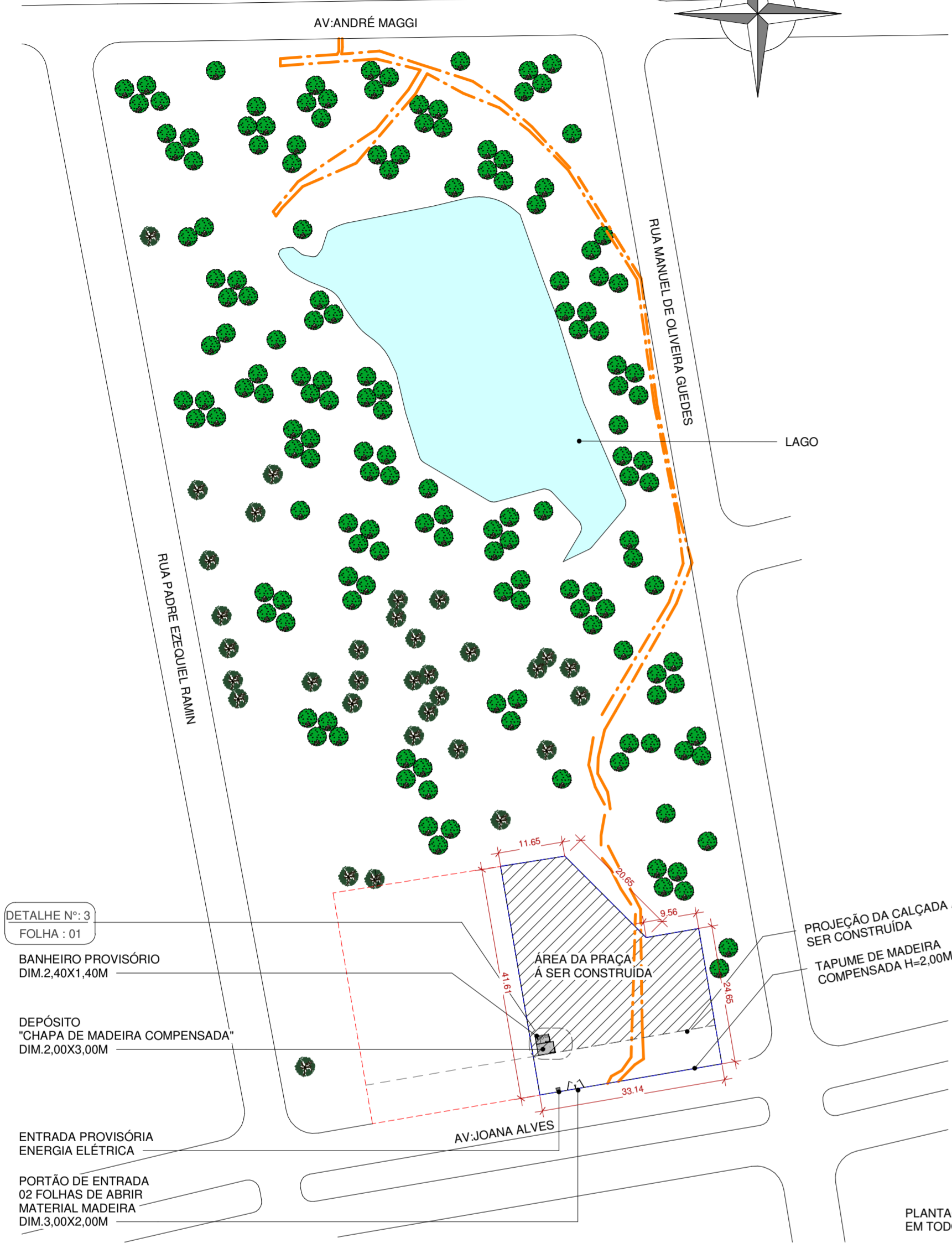
0.11 CANTEIRO DE OBRA 1 : 750
