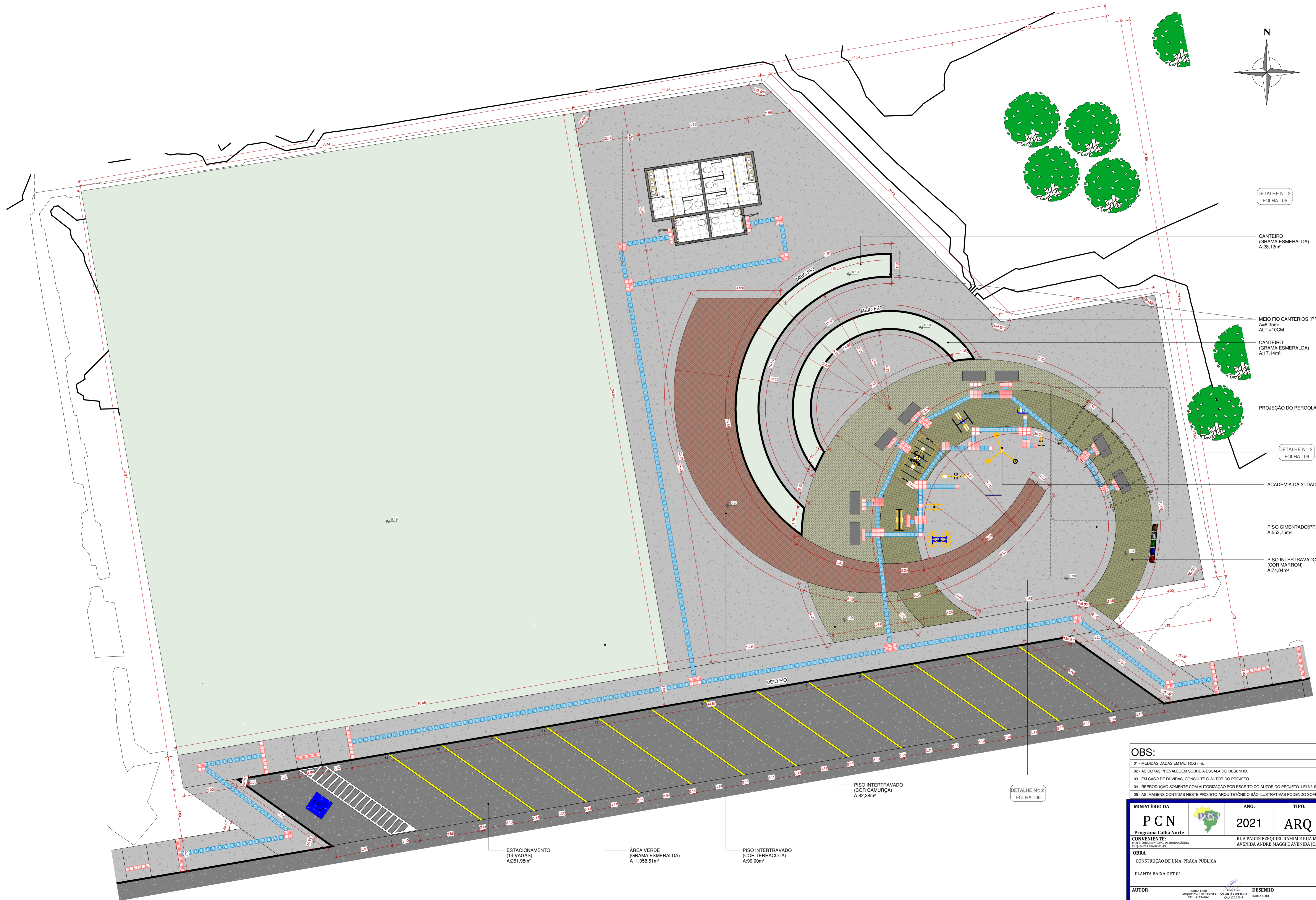
0.11 PLANTA BAIXA - DET.01 1:100
