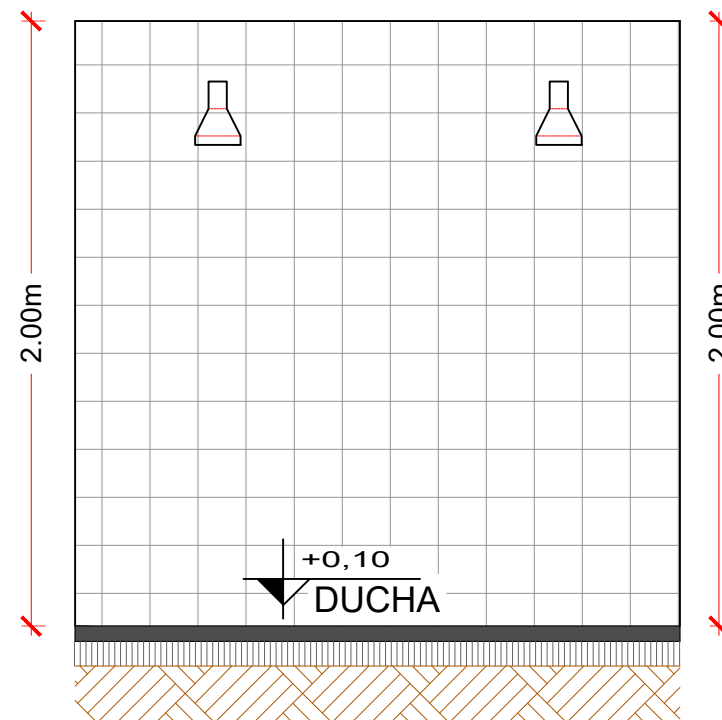
5 CORTE AA E = 1 : 25
