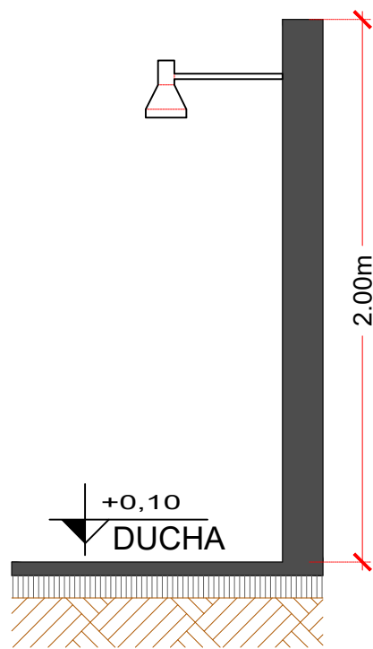
4 CORTE BB E = 1 : 25
