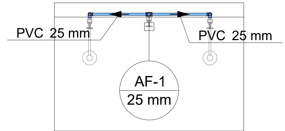
3 HIDRÁULICO E = 1 : 25
