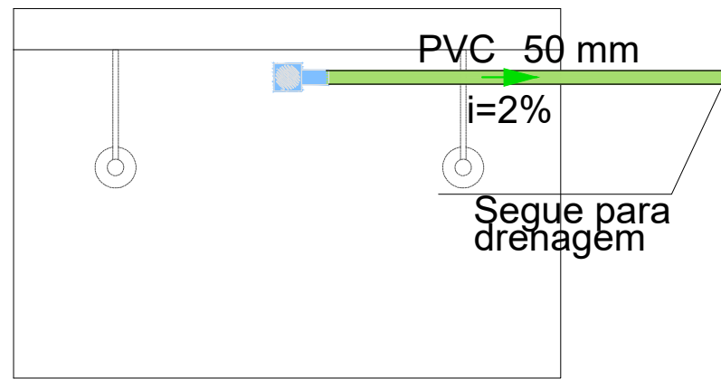
2 SANITÁRIO E = 1 : 25
